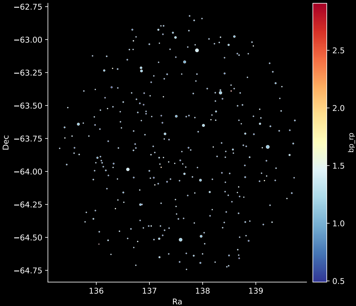
GALAH DR4 Field: [7005] Stars: 299
